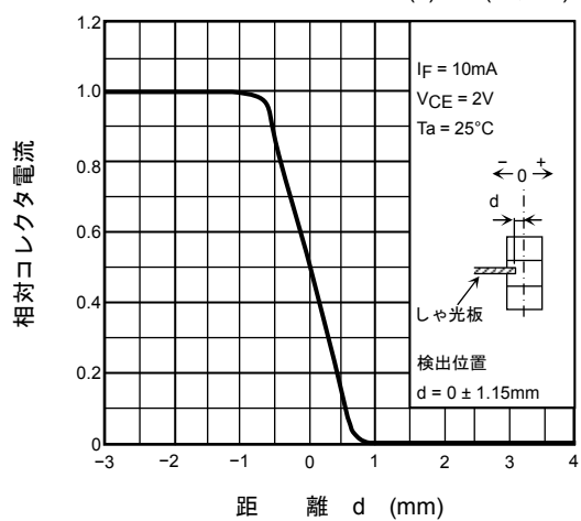
検出位置特性 (1) (代表値)
