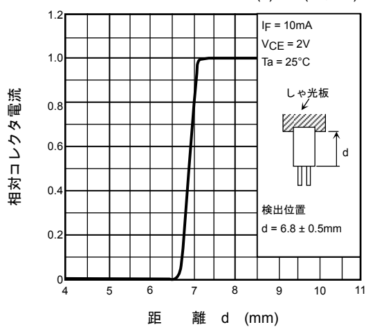
検出位置特性 (2) (代表値)
